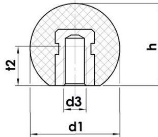
Form E mit eingefügter Gewindebuchse
