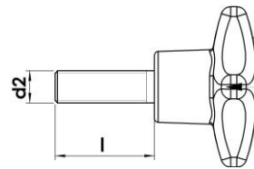
Form B mit eingefügtem Gewindebolzen (entspricht DIN 6335 Form L)
